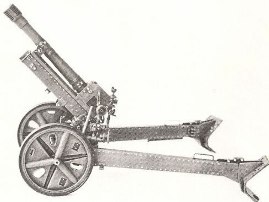
7,5 cm Gebirgsgeschütz 36 mit Metallrädern
