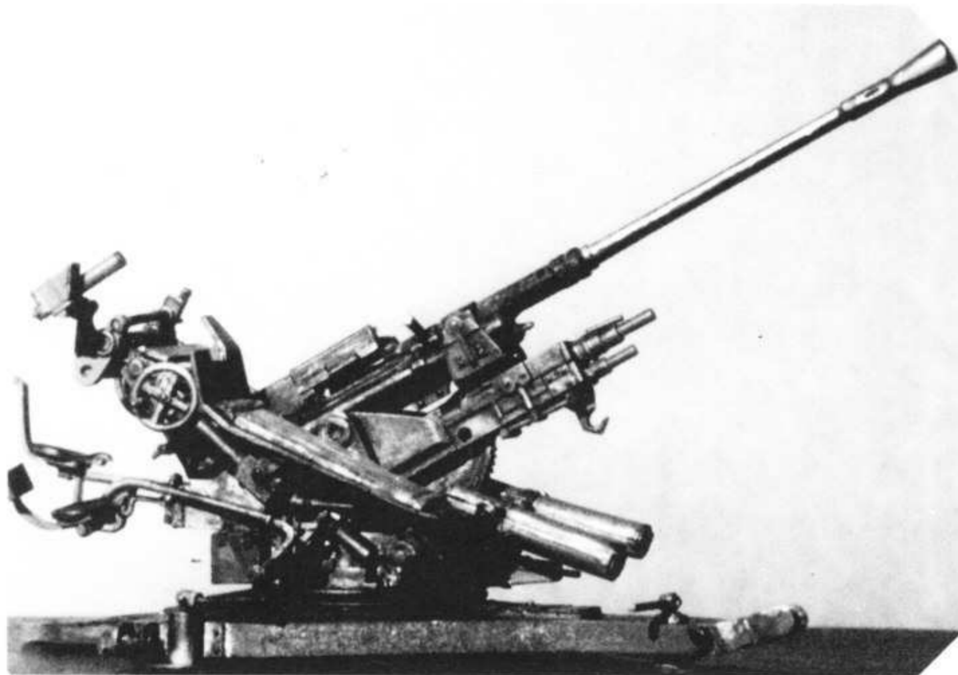
up Fl 4 3,7 cm Flak 36
