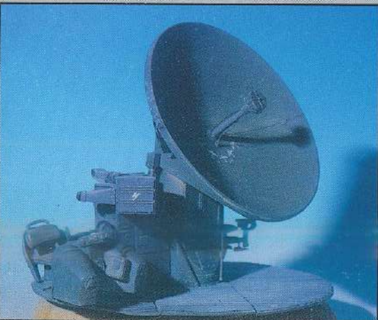
FL 41 Funkmeßgerät Würzburg 39T
