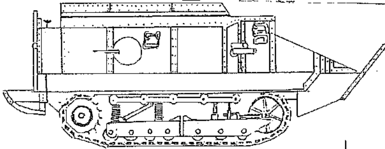
23/04 SCHNEIDER M 16
