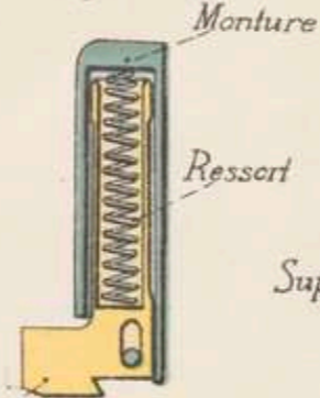
Coupe AB
