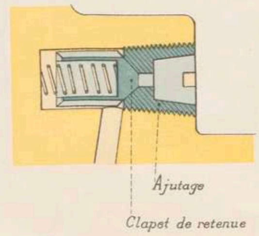
Détail d'un trou graisseur
