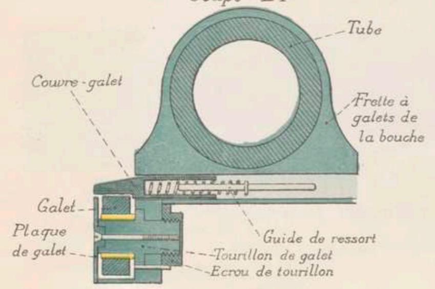
Coupe EF
