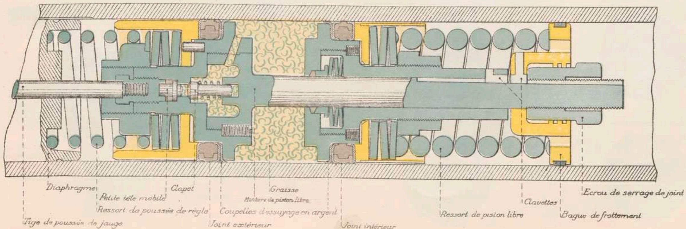
Piston libre
