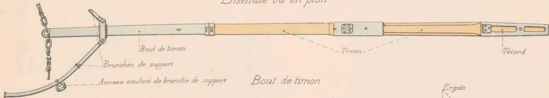
Ensemble vu en plan
