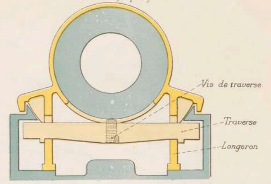
Coupe CD (v. pl. I.)
