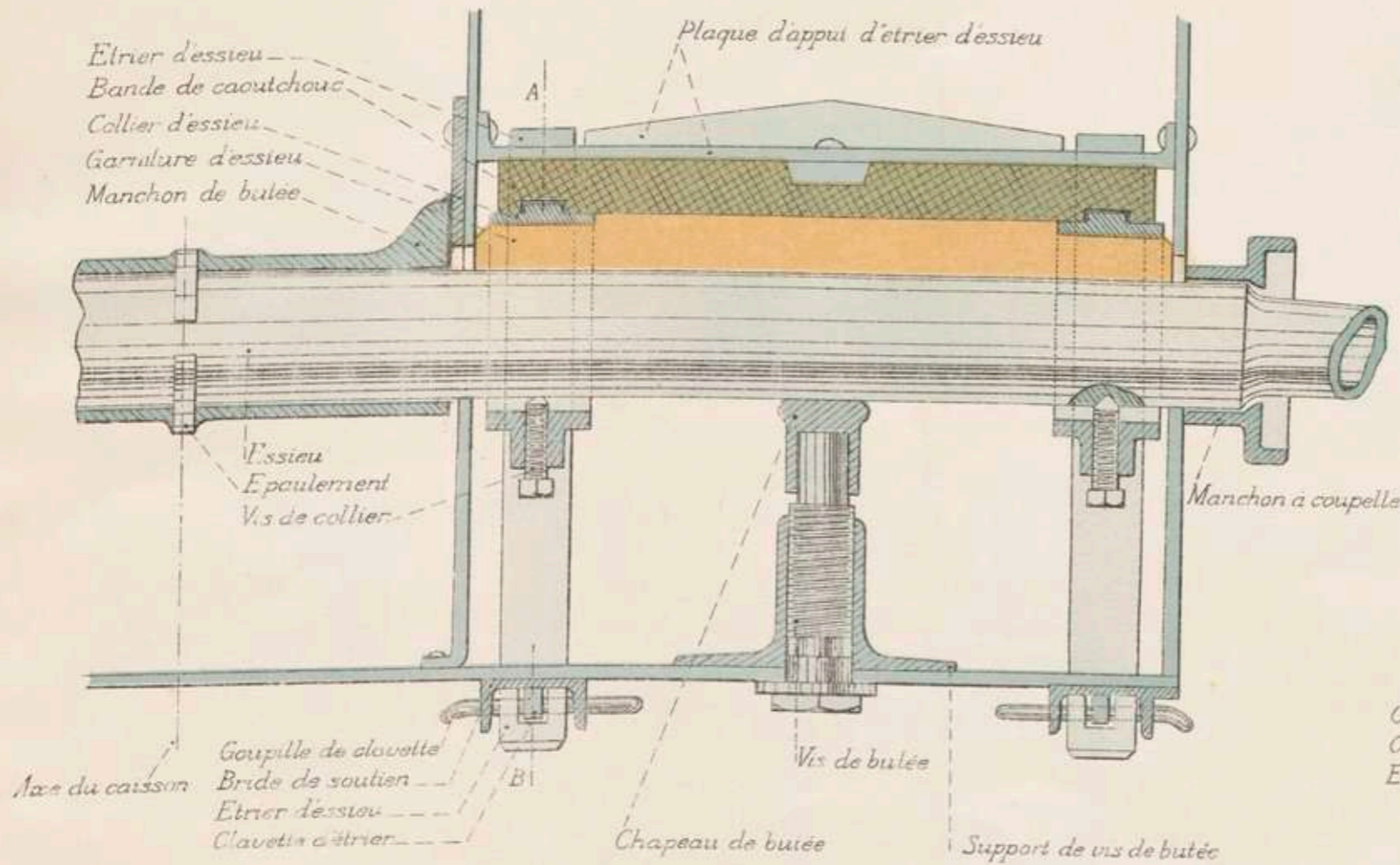
Coupe par l'axe de l'essieu
