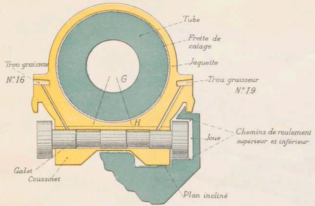
Coupe AB (v. pl. I.)
