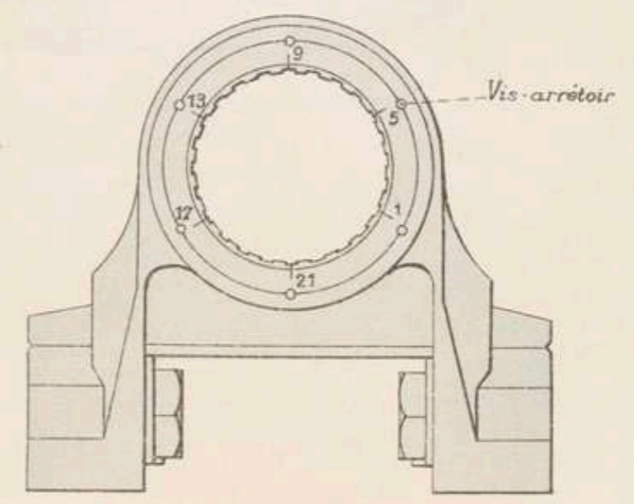
Vue avant Numérotage des rayures
