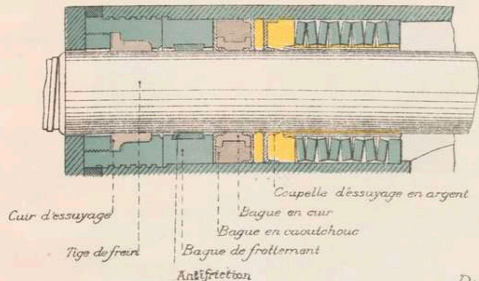
Joint arrière de tige de frein
