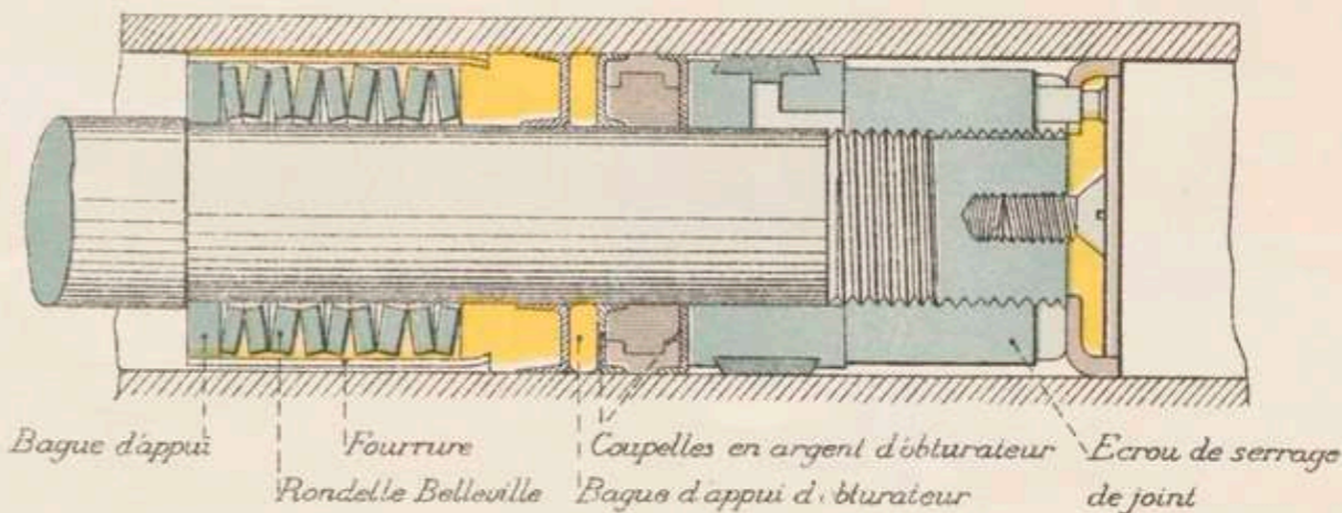
Piston de tige de frein
