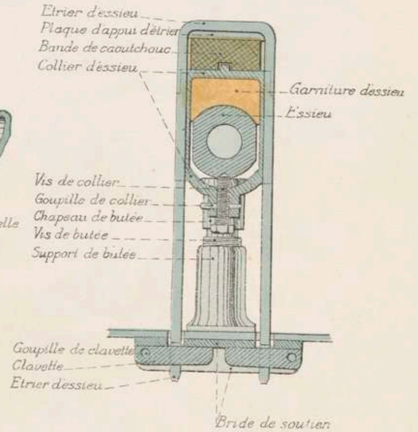
Coupe AB
