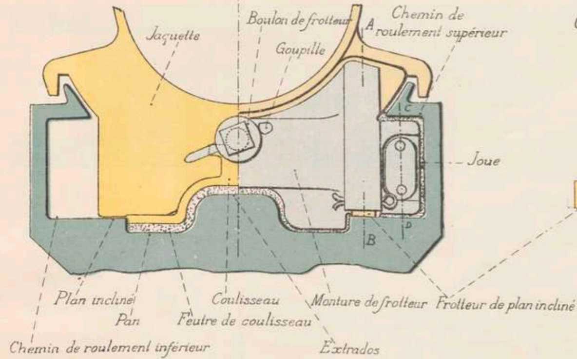
Coupe par la tranche antérieure du coulisseau
