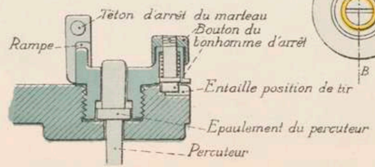
Pièce de sûreté Coupe CD - Position de tir
