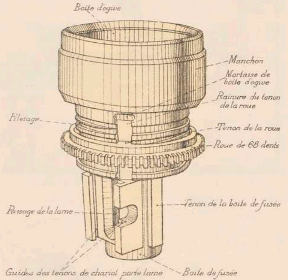
Liaison de la boîte d'ogive et de la roue de 68 dents
