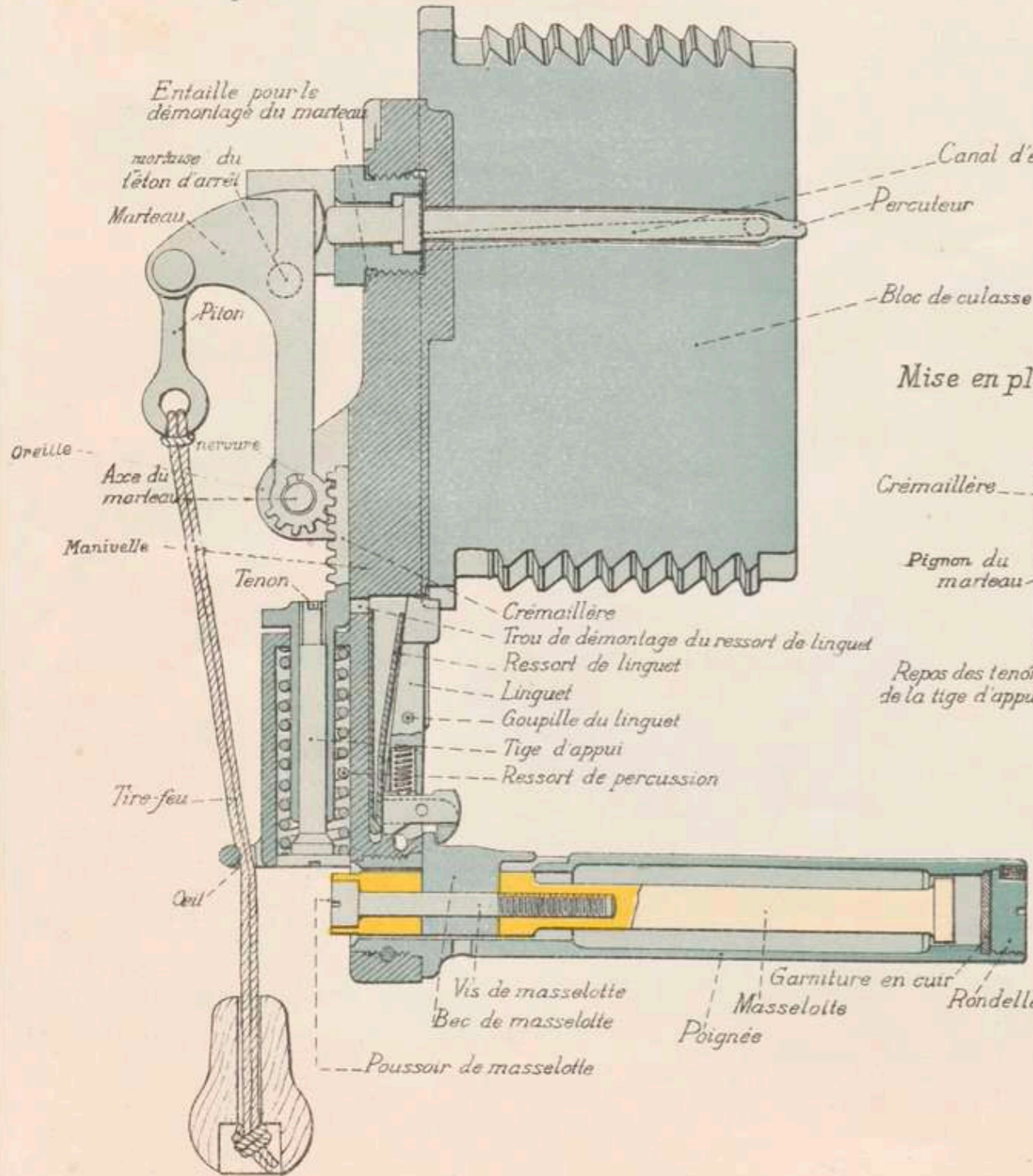
Coupe AB
