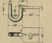
Gancho de suspension de cadena de rastra.
