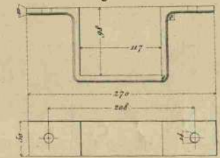
Sotabraça de brançal.
