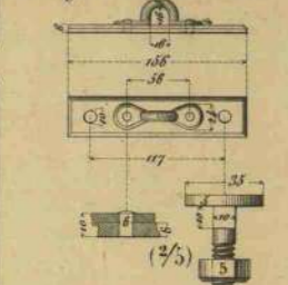
Grapa de sujecion.
