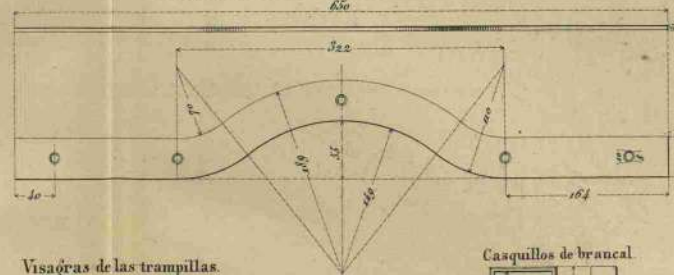
Visagras de las trampillas.
