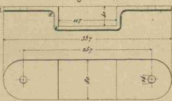
Sotabraça de vigueta.
