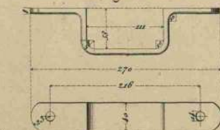
Sotabraça de telera.
