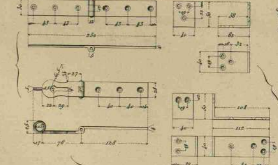
Herrajes de las cajas de espoletas y llaves.
