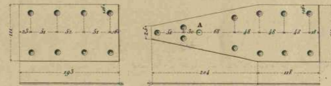
Chapas del suplemento de porta-rueda.
