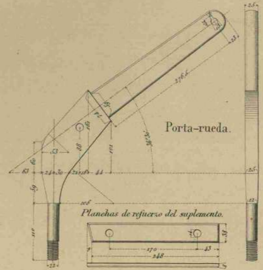
Chapas del suplemento de porta-rueda.
