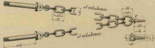
Rozaderos.
