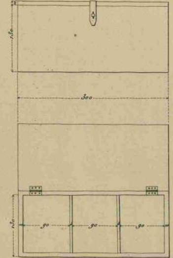
Cajita para tornillos de madera y puntas de Paris
