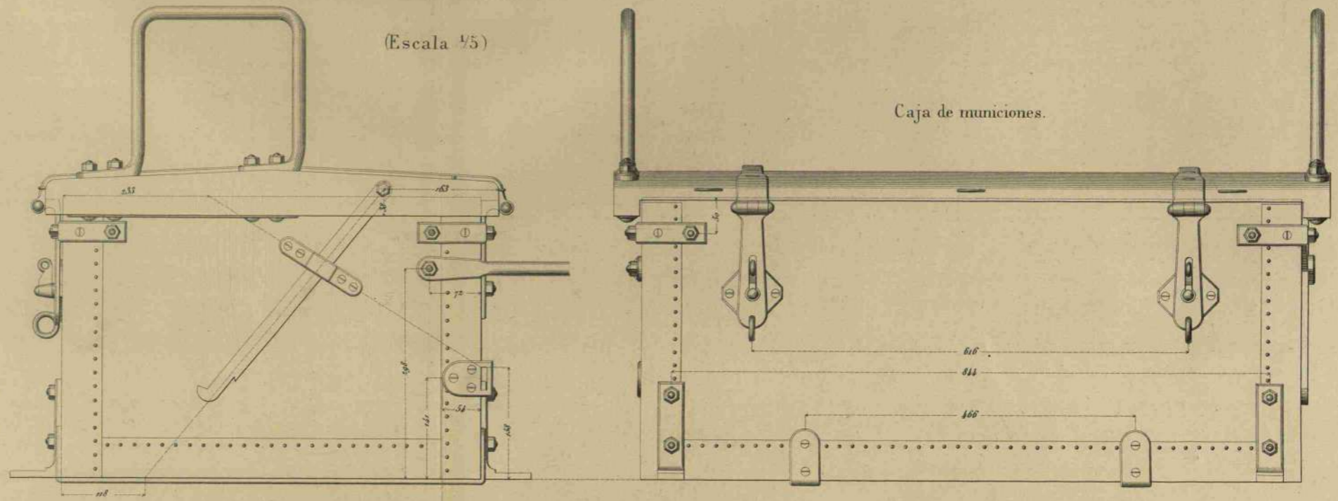
Corte de la caja por AB.
