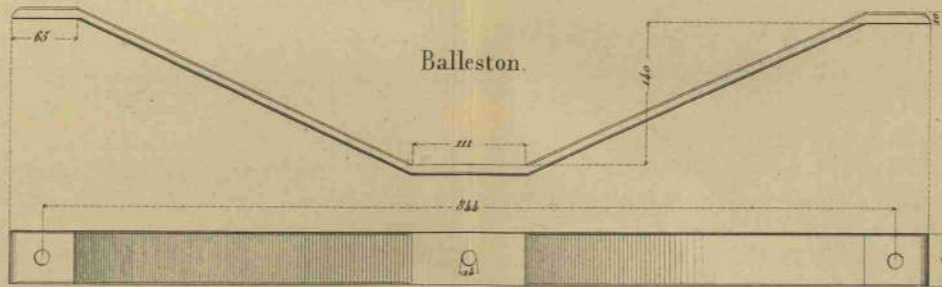
Abrazadera de suspension de la lanza de respeto.
