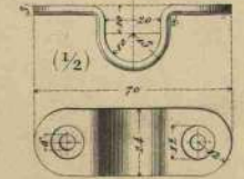
Grapas de varal.
