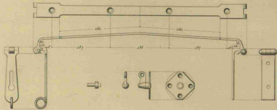
Visagras de caja de municiones.
