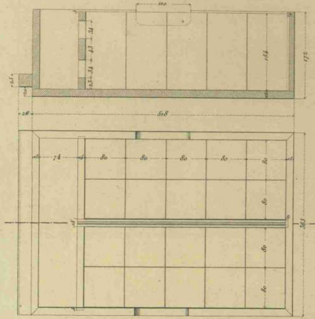
Cajas para cartuchos.
