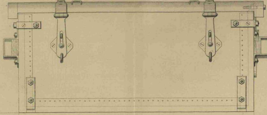
Caja para herramientas. \frac{1}{5}
