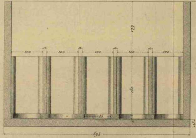
Corte de la caja por AB.
