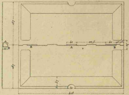
Tapa de zinc para las cajas de cartuchos.
