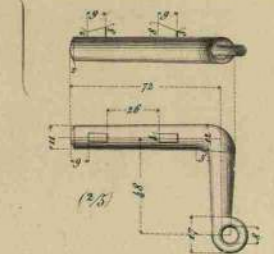
Volandera y llave del Porta-rueda.
