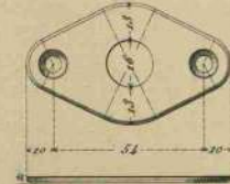
Ovahllos y perno pasador para sujetar el mástil de respeto.
