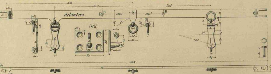
Puentes de sujecion de varal con cerraderos y anillas.
