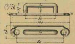
Grapa de sujecion.
