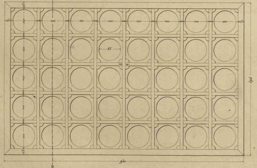
Corte de la tapa de la caja.
