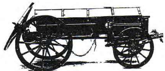
Preußischer Patronenwagen C16 1816 - 1872 Nr. 12 S
