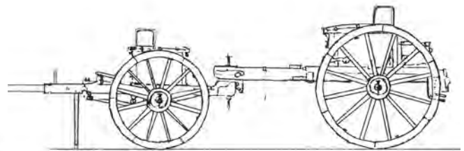
Preußischer Munitionswagen C/42/61/64 1842 Nr. 16 S
