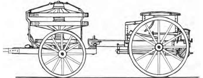
Preußischer Vorratswagen C/42 1842 Nr. 20 S
