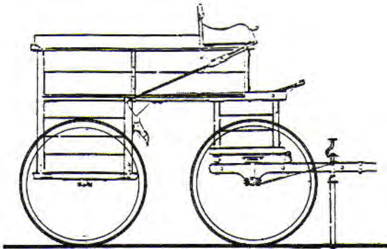
Preußischer Truppen-Medizin-Wagen 1870 Nr. 1 S
