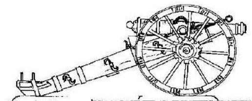
G 2591/11 - Österr. 6-Pfünder (auch für Preußen verwendbar) Gr141/91
