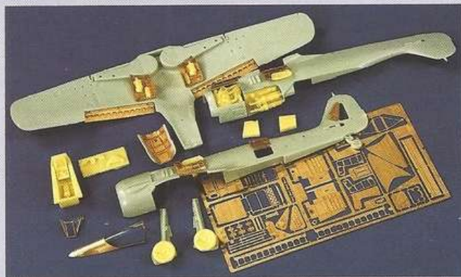
N°0831 FW-190 A8 Update Set (Hasegawa) 1:72
